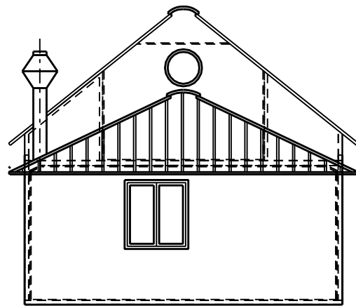
VISTA B
